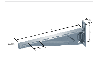
CE ESCR Escuadra soporte reforzada coliso
