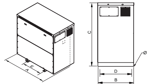
Desde 500 kVA
