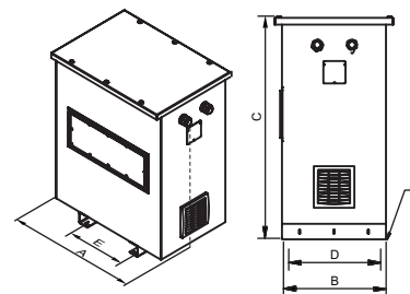
Desde 80 kVA
