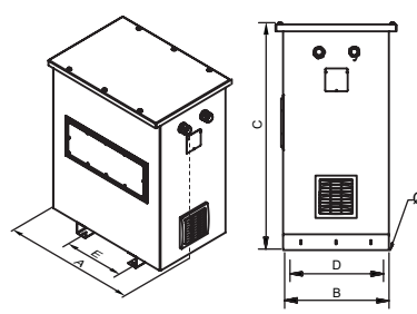
TTFZ IP54
