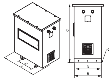
Desde 40 kVA
