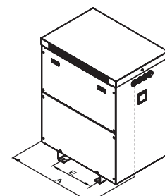
Desde 31,5 kVA
