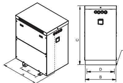
Desde 25 kVA
