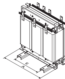
Desde 200 kVA
