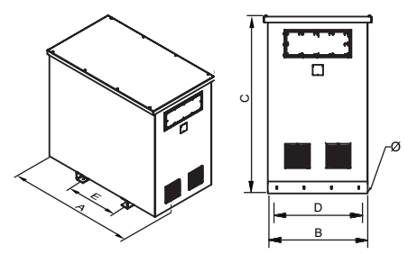
TTFZ IP54
