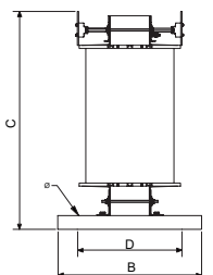
Desde 63 kVA
