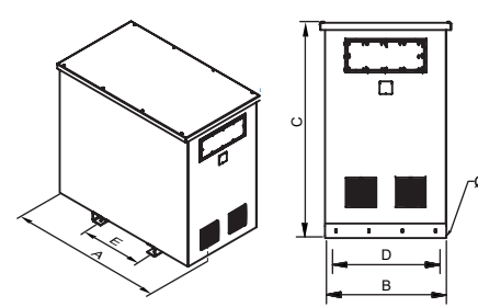
Desde 500 kVA
