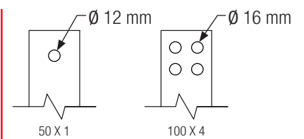
Conexión pletina
