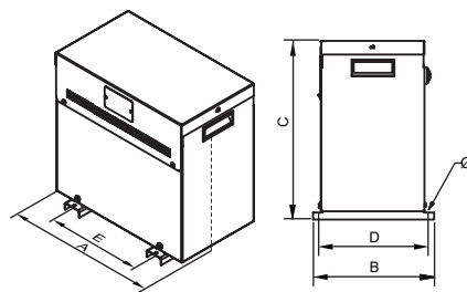
THW IP23
