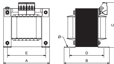
Desde PXR315
