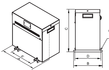
Hasta 5 kVA
