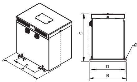
Hasta 3,15 kVA
