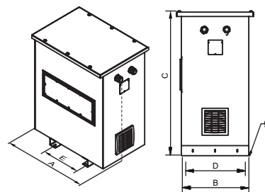
Desde 25 kVA
