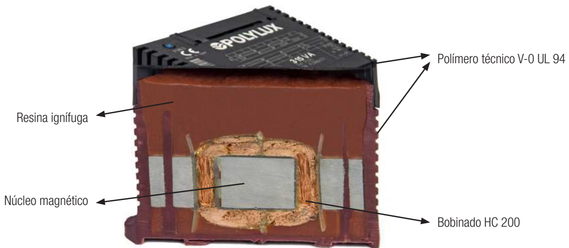
Transformador seccionado
