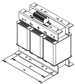
Hasta 3,15 kVA
