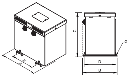
Hasta 2 kVA
