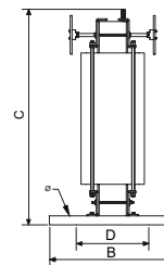
Desde 200 kVA
