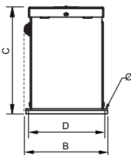
Hasta 2 kVA
