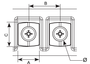
Borne M5
