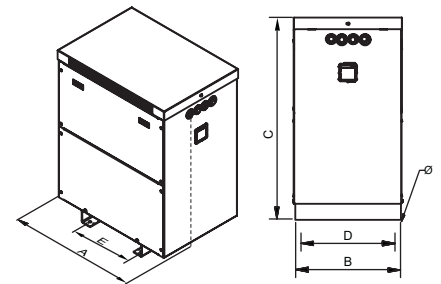
Desde 31,5 kVA
