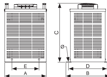
Desde PD3150
