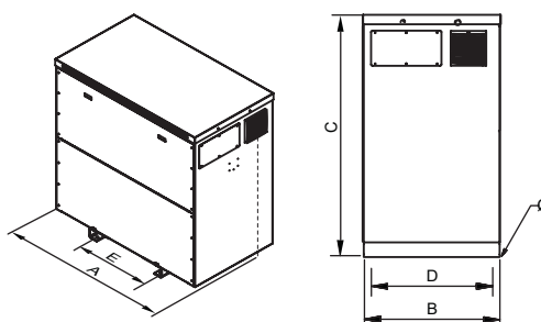
Desde 500 kVA
