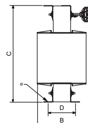
Desde 31,5 kVA
