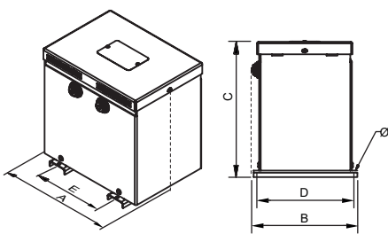
Hasta 2 kVA
